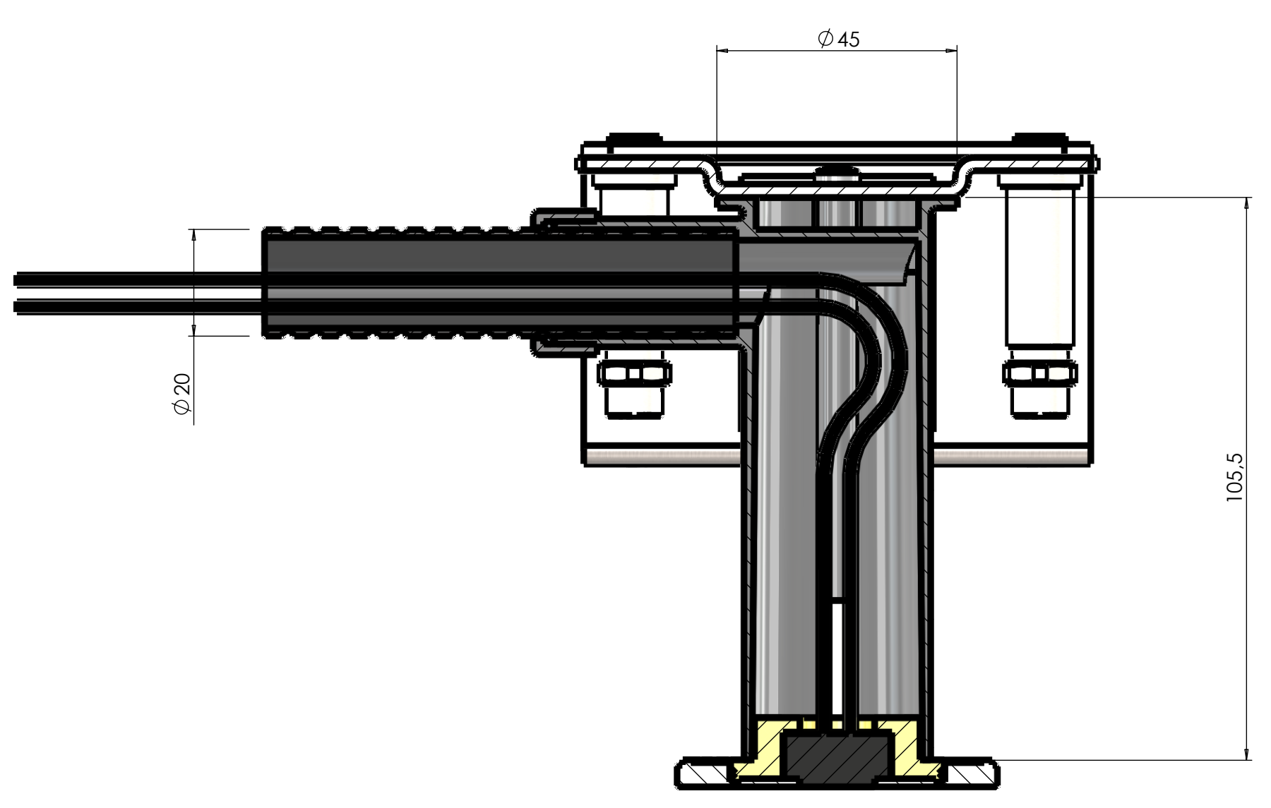
SEZIONE B-B
